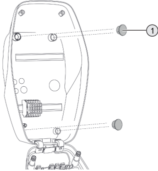
7. Ábra: Záródugók
