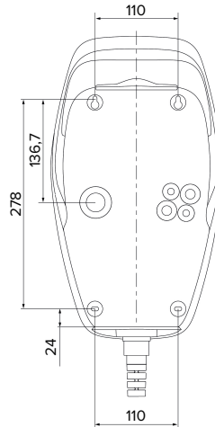
Εικ. 6: Διαστάσεις διάτρησης [mm]
