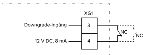
Fig. 14: Principkopplingschema: Anslutning av en extern brytarkontakt (standardinställning: NO)
