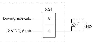
Kuva 14: Periaatekytkentäkaavio: ulkoisen kytKentäkontaktin liitäntä (vakioasetus: NO)
