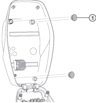
Kuva 7: Sulkutulpat
