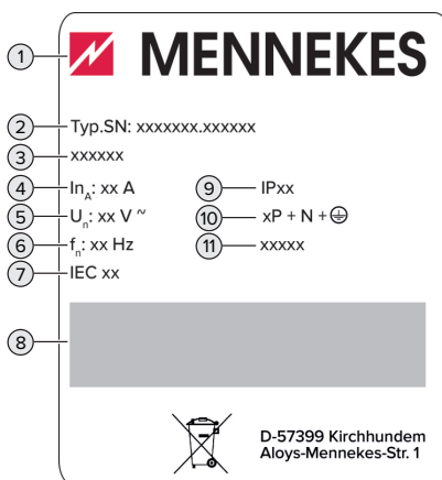
Fig. 1: Produkttypeskilt (eksempel)
