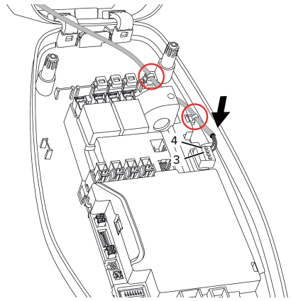
Afb. 13: Aansluiting downgrade-ingang
