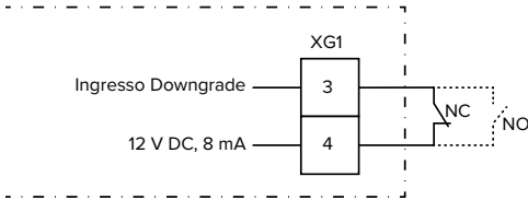
Fig. 14: Schema di principio: collegamento di un contatto di commutazione esterno (impostazione di default: NO)
