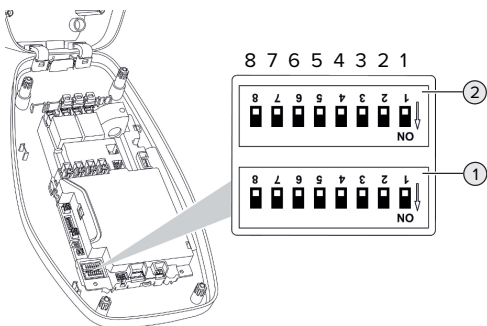
Afb. 12: Dipschakelaar (uitleveringstoestand)
