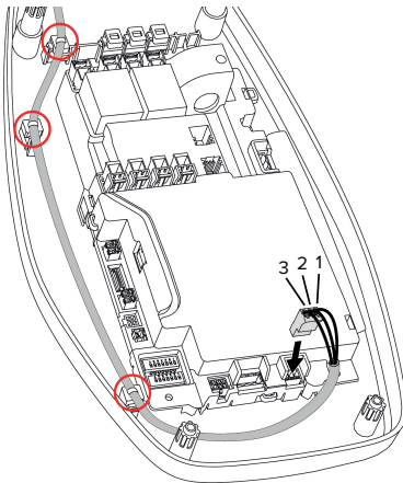
Fig. 11: Anslutning dataledning [mm]
