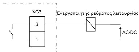
Εικ. 10: Διάγραμμα συνδεσμολογίας: Σύνδεση εξωτερικού ενεργοποιητή ρεύματος λειτουργίας
