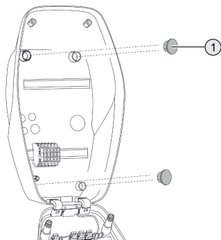
Fig. 7: Lukkepropper
