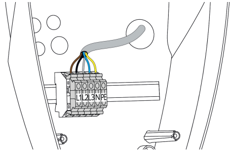
Kuva 8: Jännitesyötön liitäntä
