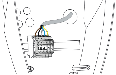
8. Ábra: Feszültségellátás csatlakoztatása
