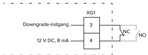
Fig. 14: Principskema: Tilslutning af en ekstern om-skifterkontakt (standardindstilling: NO)
