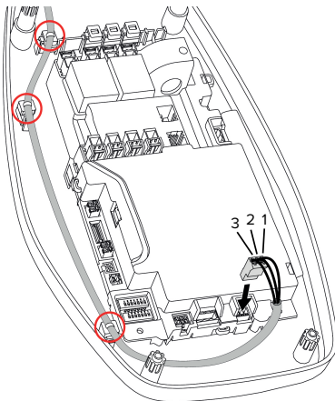
Fig. 11: Collegamento linea di trasmissione dati [mm]
