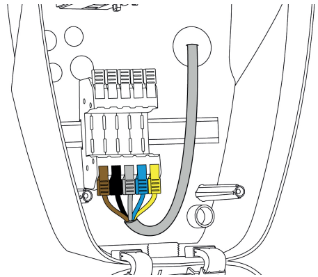
Fig. 8: Collegamento dell'alimentazione elettrica (esempio)
