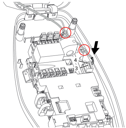
Abb. 14: Anschluss Downgrade-Eingang
