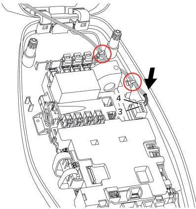
Afb. 14: Aansluiting downgrade-ingang
